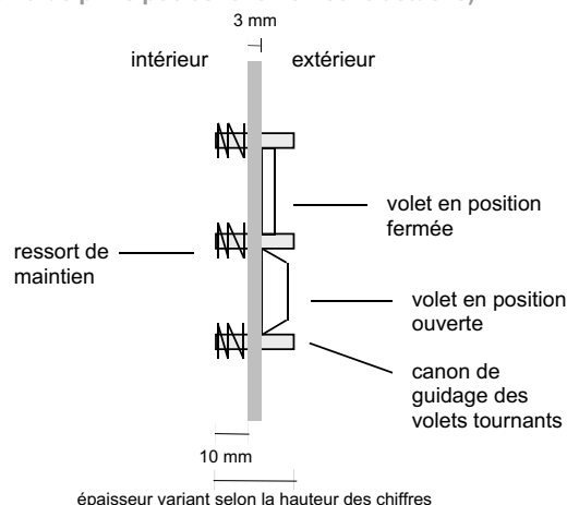
VUE DE COTE D'UNE PLAQUE (schéma de principe / échelle non contractuelle)
